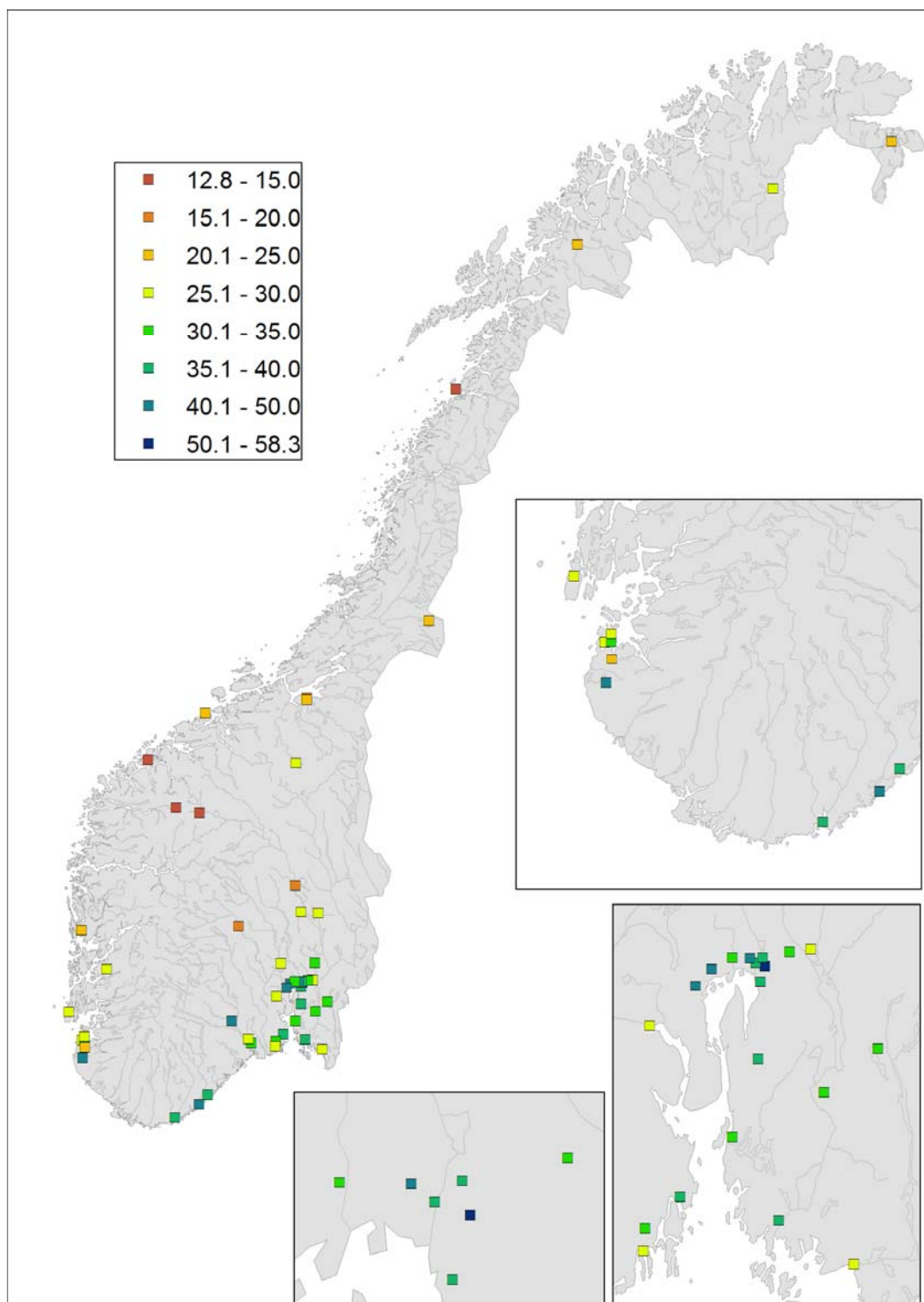
Figur 4.3 Estimert av 30 minutters nedbør (mm) med 200 års returperiode
