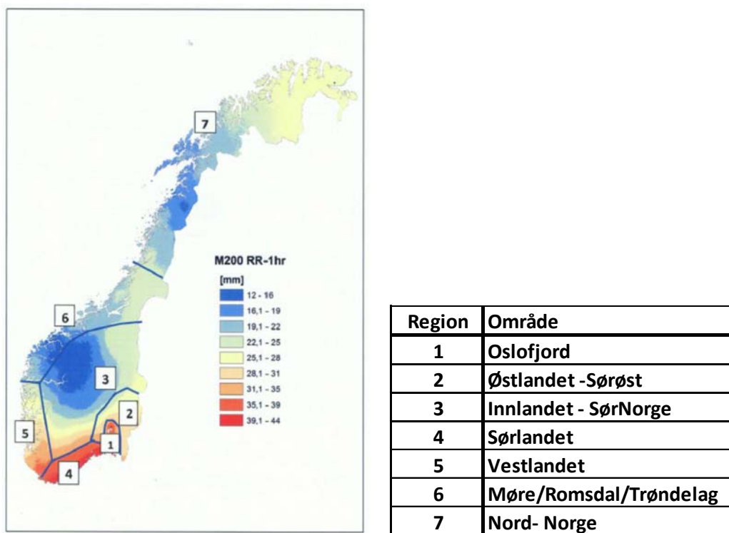
Figur 4.9. Tentativ regioninndeling av IVF-serier for 200 års returperiode
