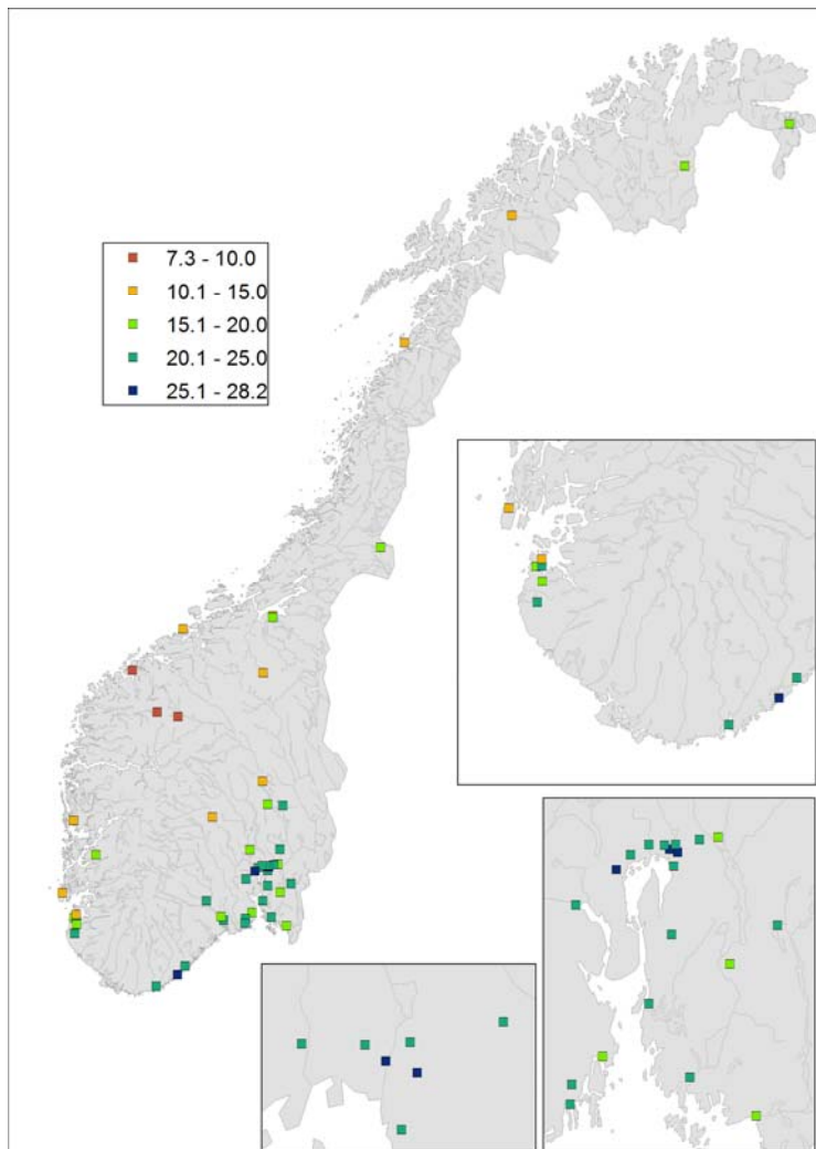
Figur 4.2 Estimat av 10 minutters nedbør (mm) med 200 års returperiode
