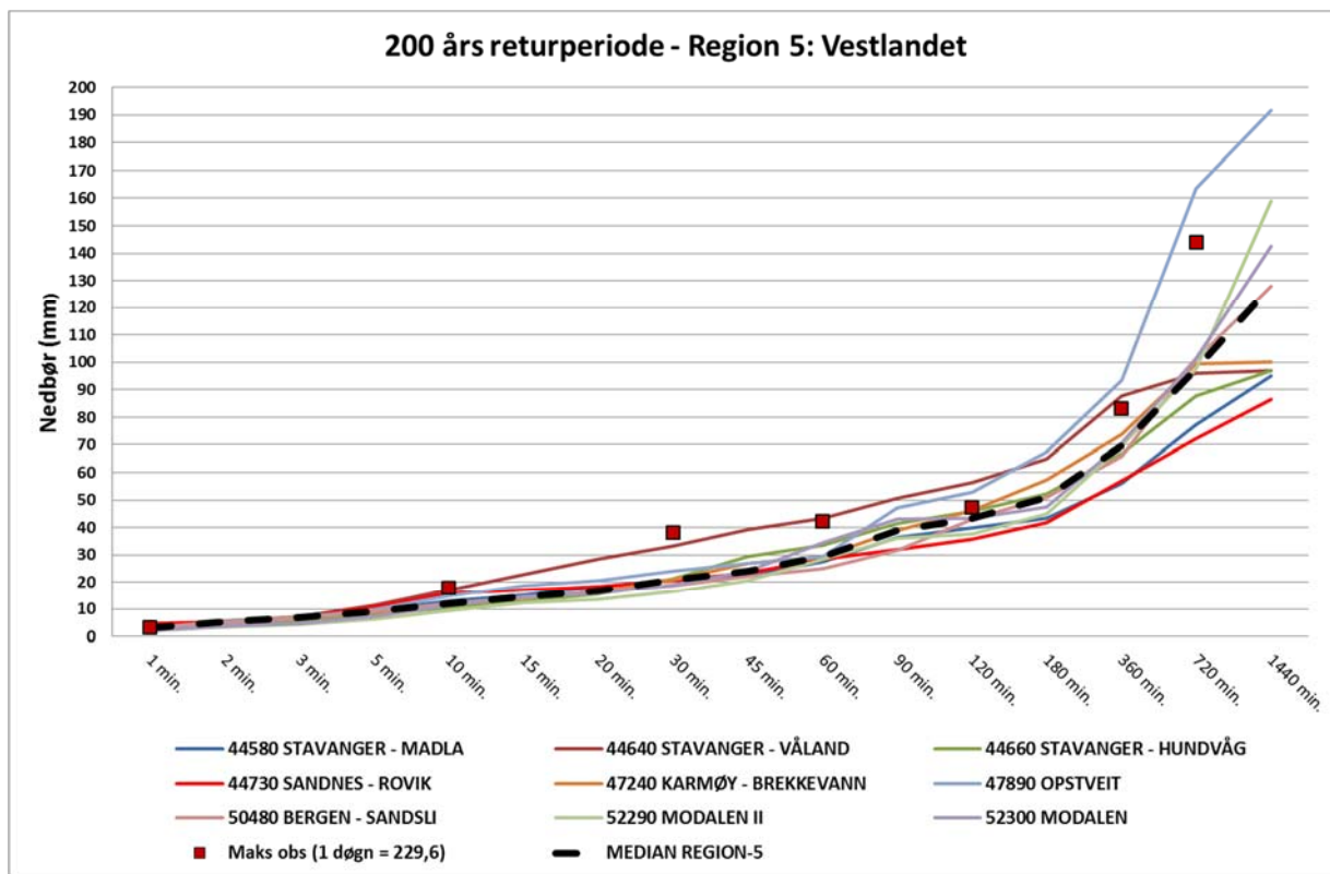
Figur 4.14 IVF-verdier for 200 års returperiode for 9 stasjoner i Region 5: «Vestlandet»
