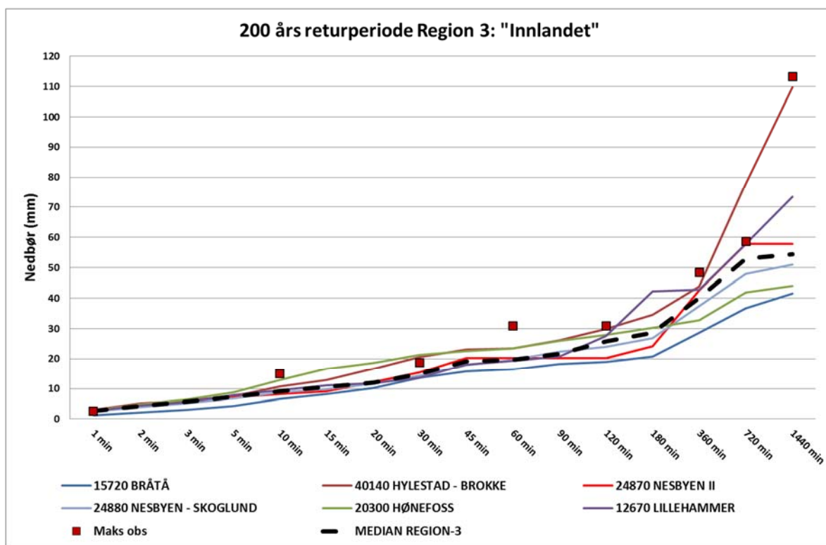
Figur 4.12 IVF-verdier for 200 års returperiode for 6 stasjoner i Region 3: «Innlandet»
