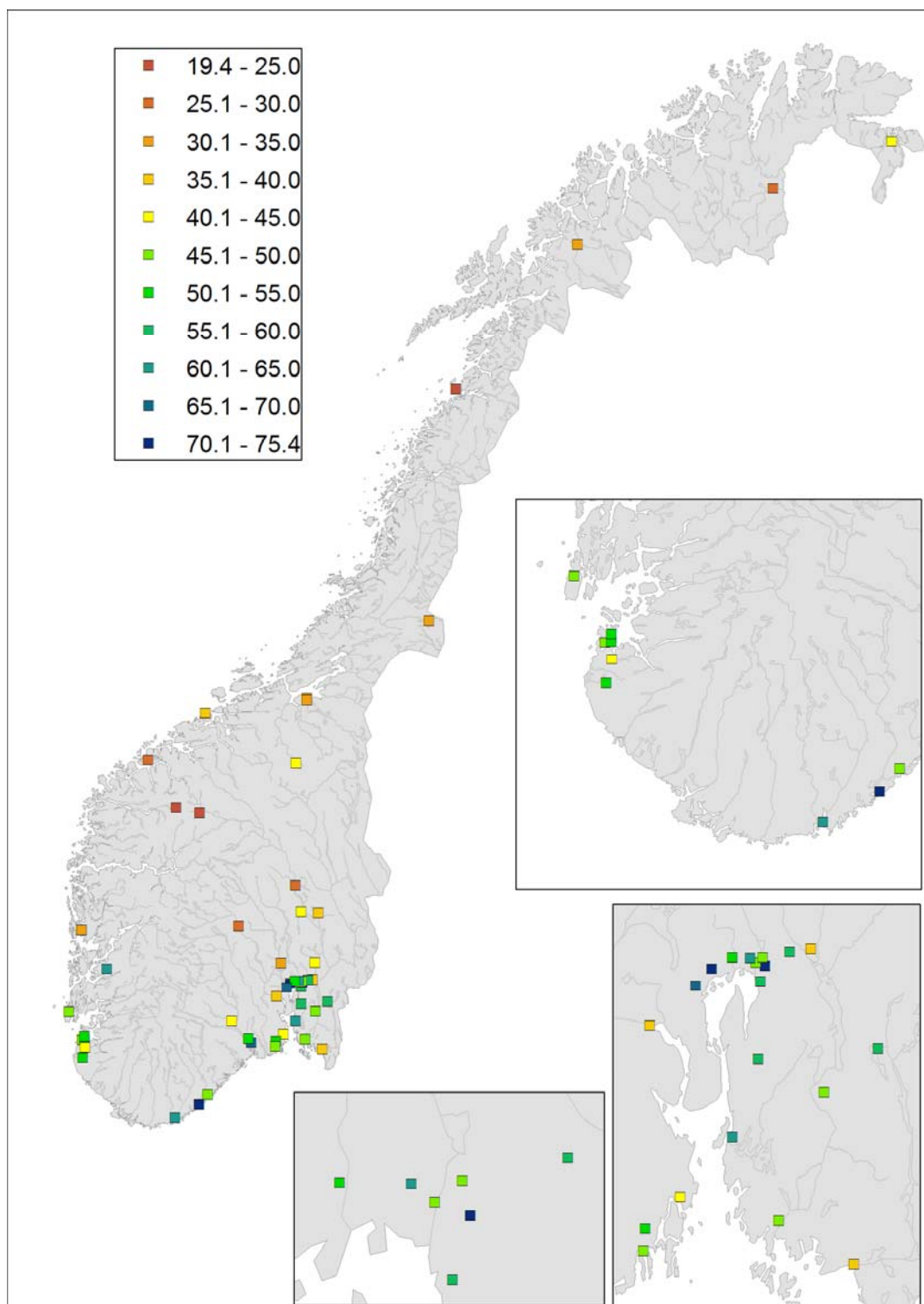
Figur 4.5 Estimert av 2 timers nedbør (mm) med 200 års returperiode
