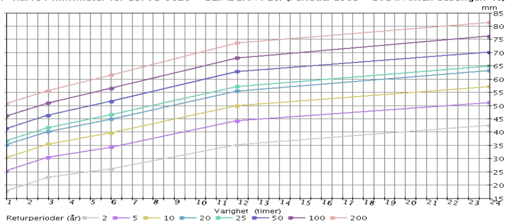
Figur 4.1b: Eksempel på IVF-kurver (i millimeter) for 18701 Oslo-Blindern (1968 - 2014) for 1 – 24 timer
