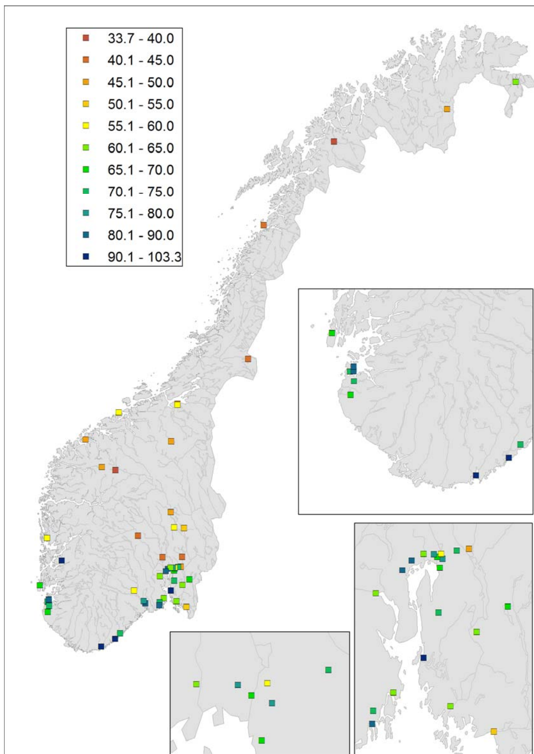
Figur 4.6 Estimert av 6 timers nedbør (mm) med 200 års returperiode
