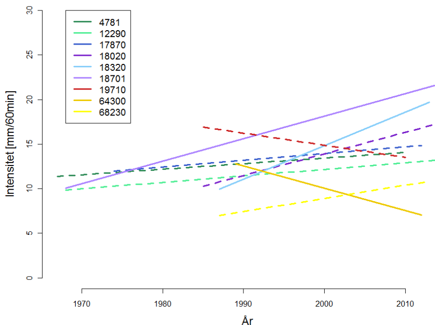
Figur 5.3 Sommernedbør i løpet av 60 min – Trend for høyeste observerte verdi per år
