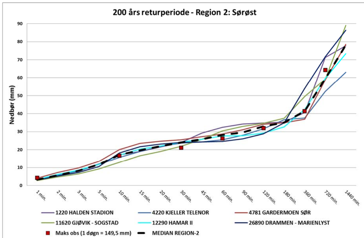
Figur 4.11 IVF-verdier for 200 års returperiode for 6 stasjoner i Region 2: «Østlandet SØ»
