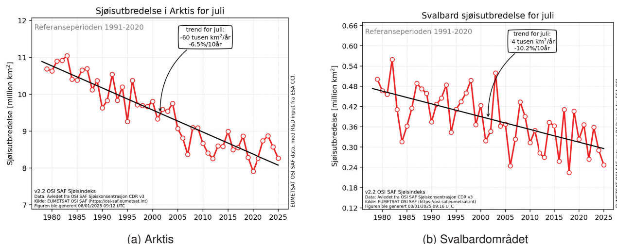
Figur 2: Sjøisutbredelsen (a) i Arktis og (b) for Svalbardområdet for juli i perioden 1979–2025. Trenden er beregnet i forhold til referanseperioden 1991–2020. Svalbardområdet er markert på kartet i figur 1.
